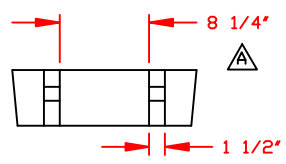
LIFTING LUG DETAIL (6) PLACES SCALE: 1'=1'-0"
