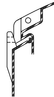
LIP DETAIL AT LUG SCALE: 1 1/2" = 1'-0"
