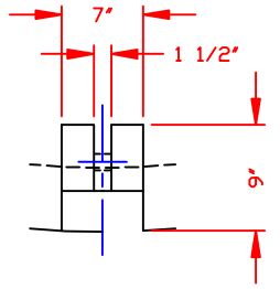
LIFTING LUG DETAIL (6) PLACES SCALE: 1"=1'-0"
